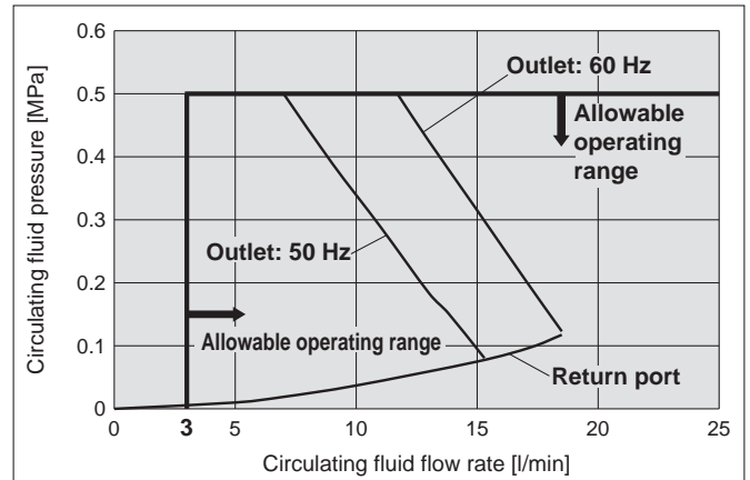
HRR012/018/024/030-□□-20-MT
