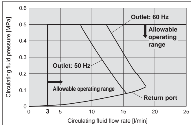
HRR012/018/024/030-□□-20-T
